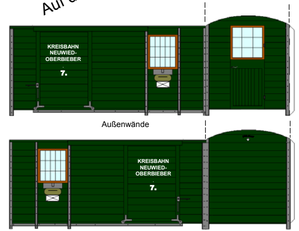
Postgepäckwagen N o . 7
