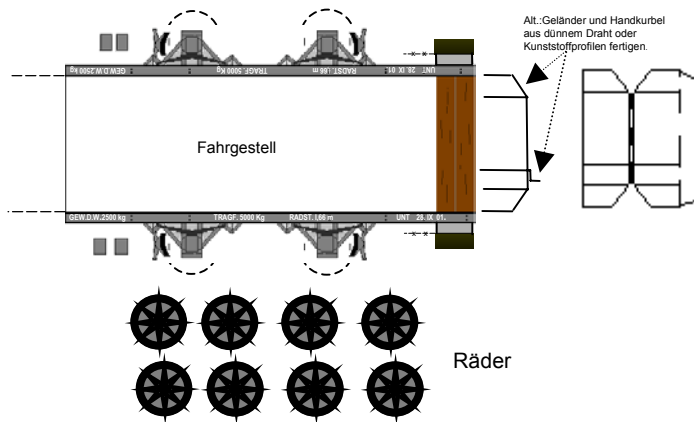
Offener Güterwagen N o . 17 mit Drehtüren
